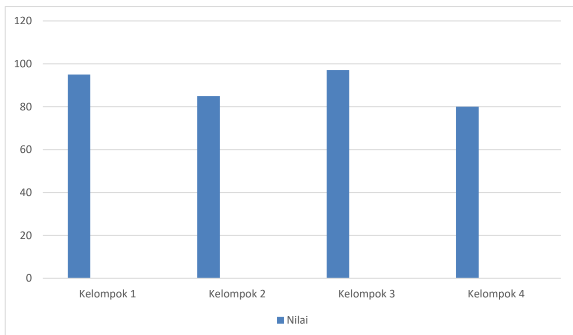
Gambar 1. diagram batang Penilaian tugas kelompok
